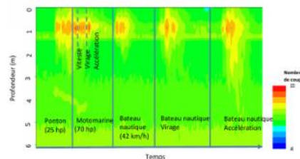
Figure 9: Zoom sur l'impact des embarcations motorisées selon différents modes de fonctionnement Lors de l'accélération la puissance des bateaux est corrélée à la profondeur impactée
